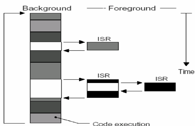
图 2-1 前后台系统
