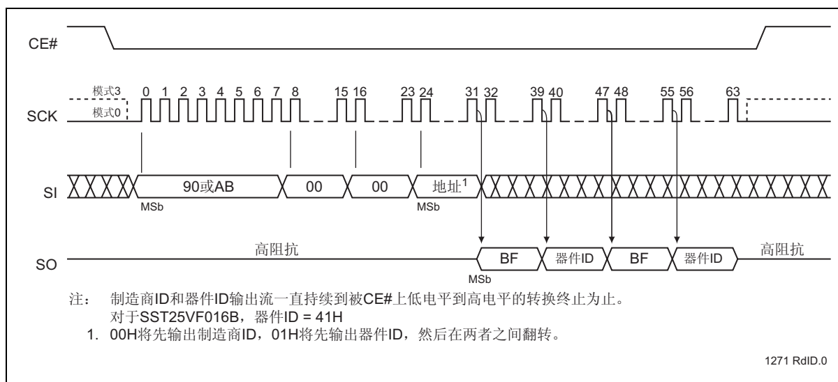
图 21: 读 ID 序列
