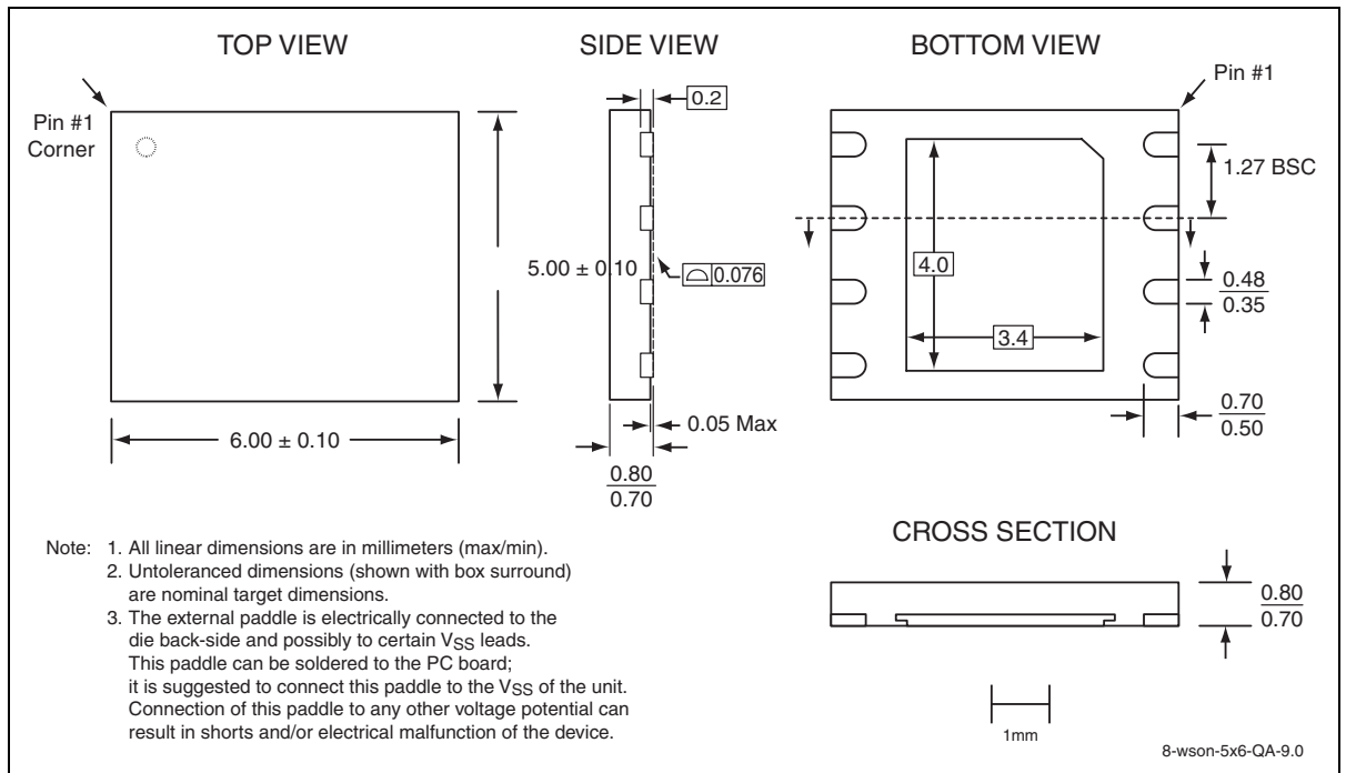
图 29: 8 触点超薄型小外形无引脚 (WSO) SST 封装代码: QA
