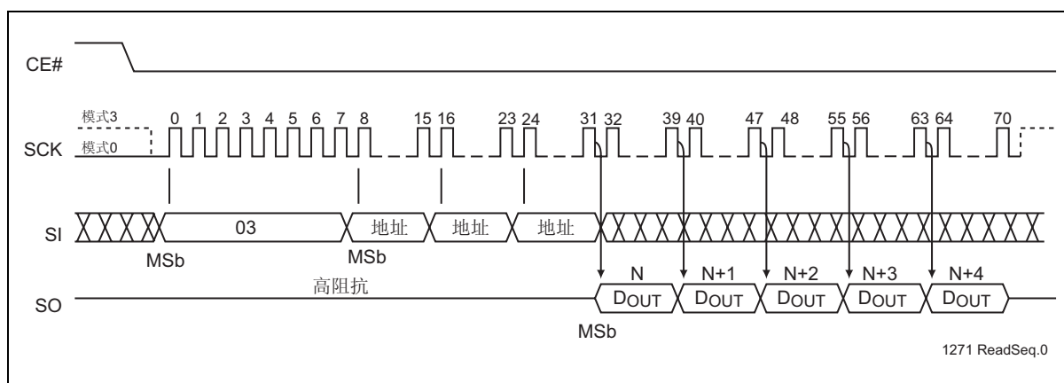
图 5: 读序列
