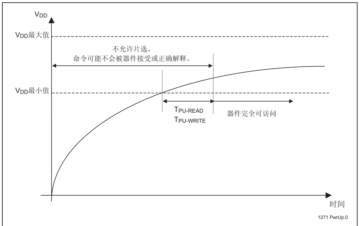
图 25: 上电时序图
