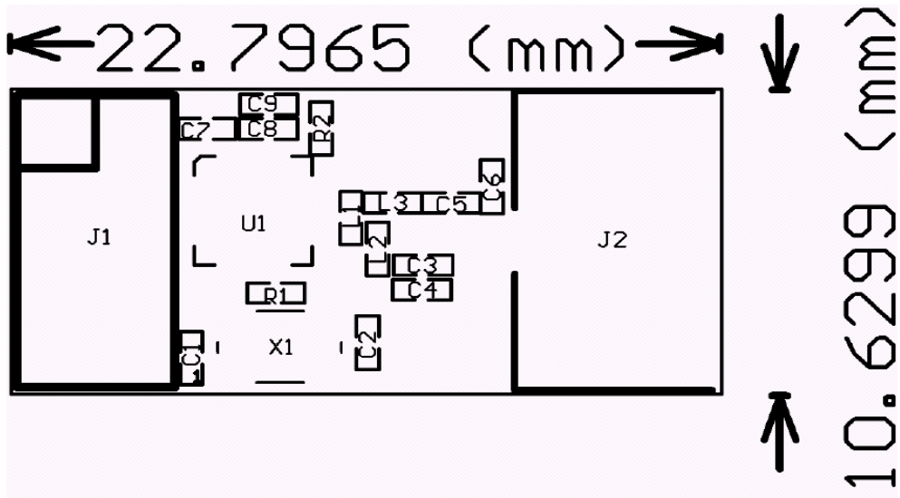
顶层丝印层
