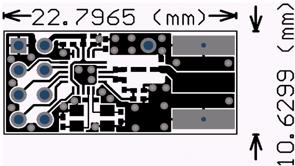
顶层布线
