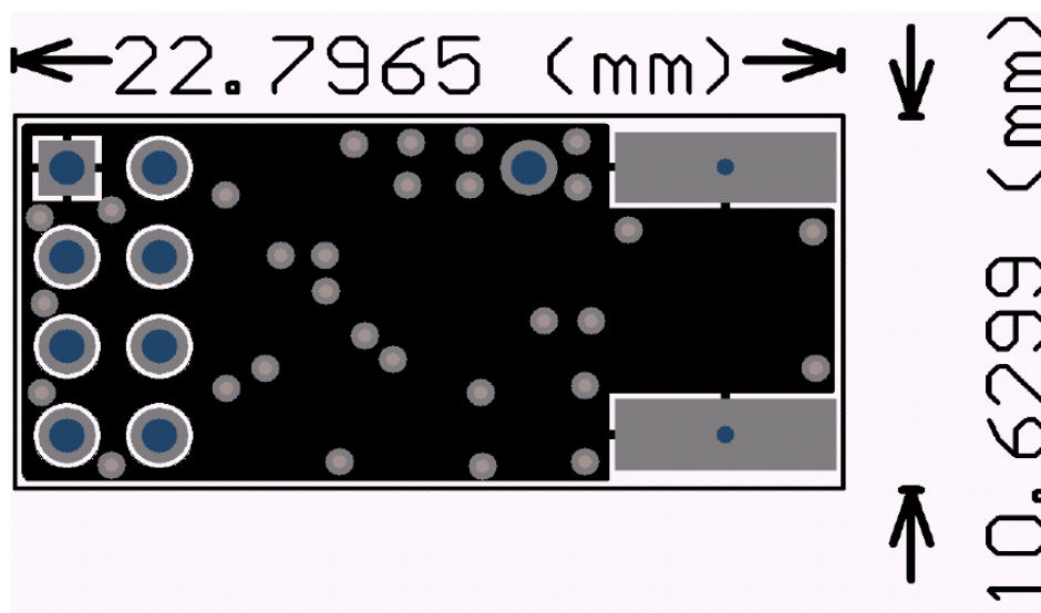
底层布线
