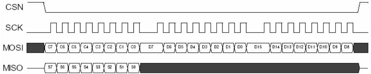
图 9、SPI 写操作
