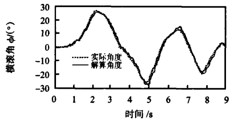
图 4 横滚角
