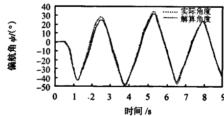
图 5 偏航角
