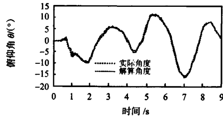
图 3 俯仰角
