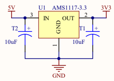
系统供电稳压
