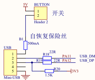
供电、开关及usb-hid
