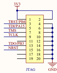
调试JTAG、SWD接口
