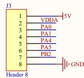
通用I/O接口
