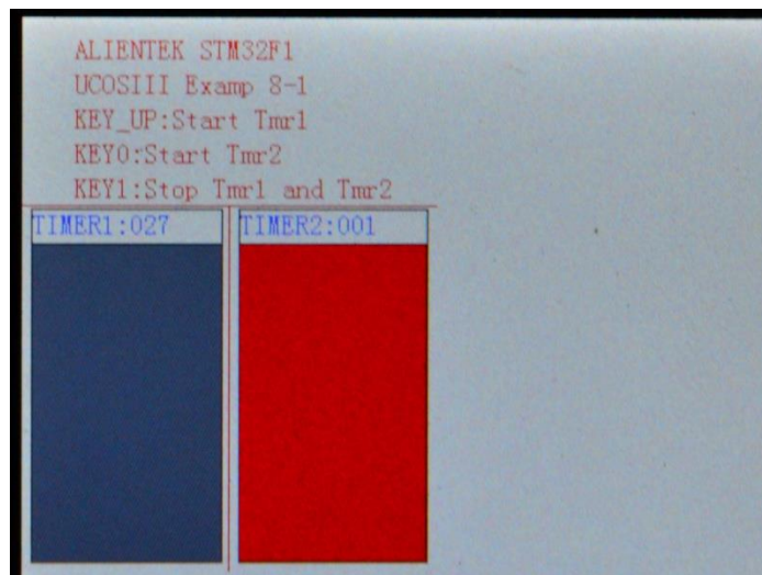
图 8.2.3 开启定时器 2 后的 LCD 界面。
