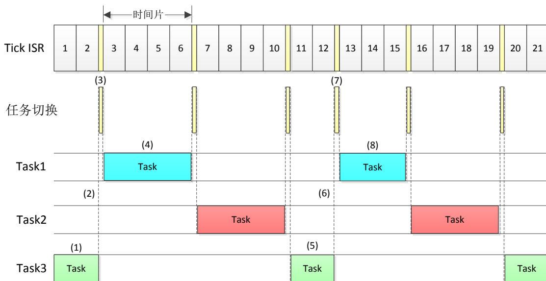
图 5.6.1 轮转调度
