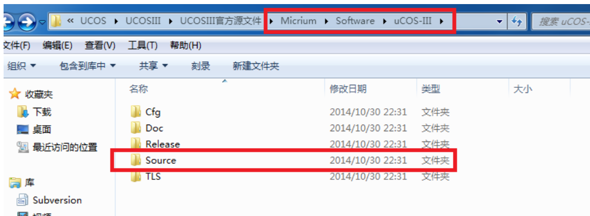
图 4.2.2 UCOSIII 3.03 源码
