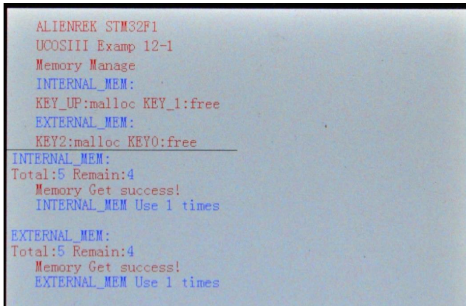
图 12.4.3 申请内存
