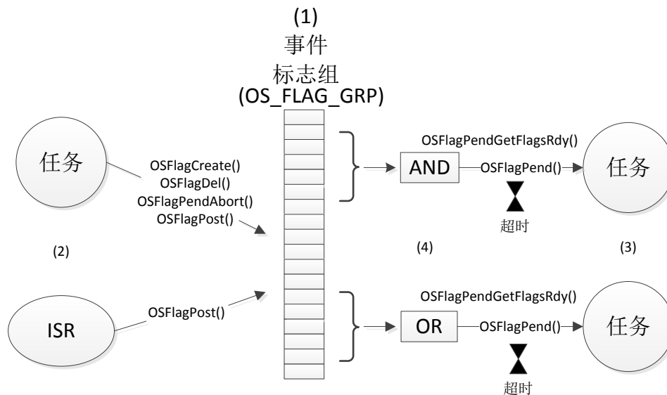
图 11.1.1 事件标志组
