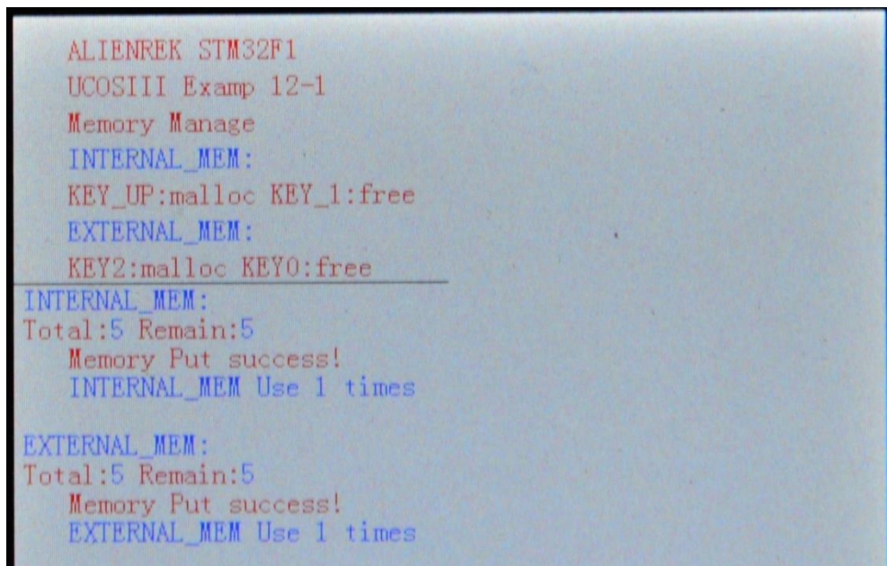
图 12.4.4 释放内存
