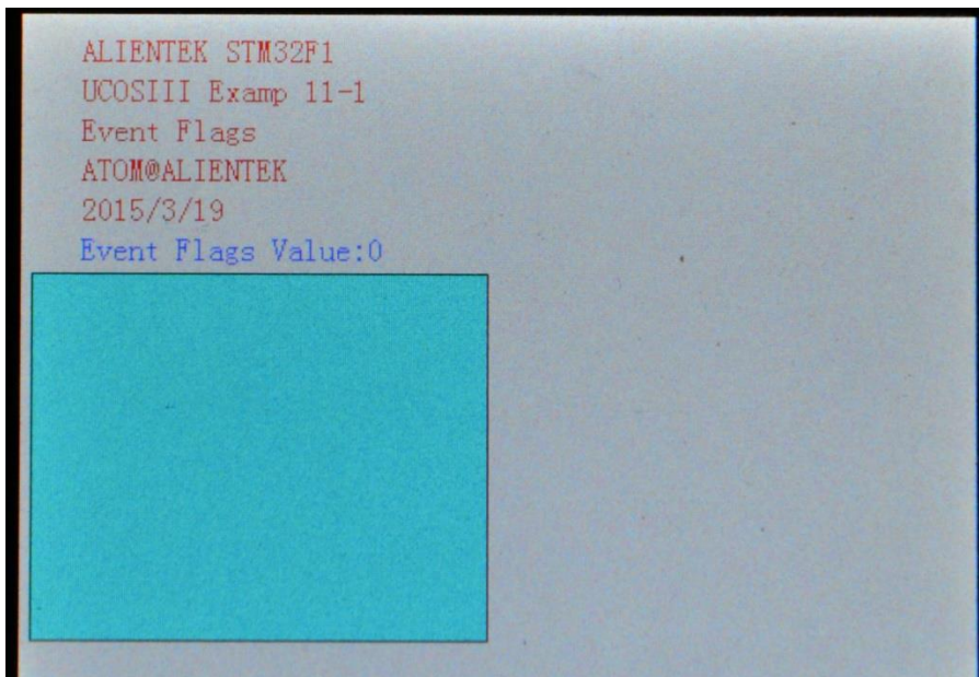
图 11.3.3 按下 KEY1 后的 LCD 界面
