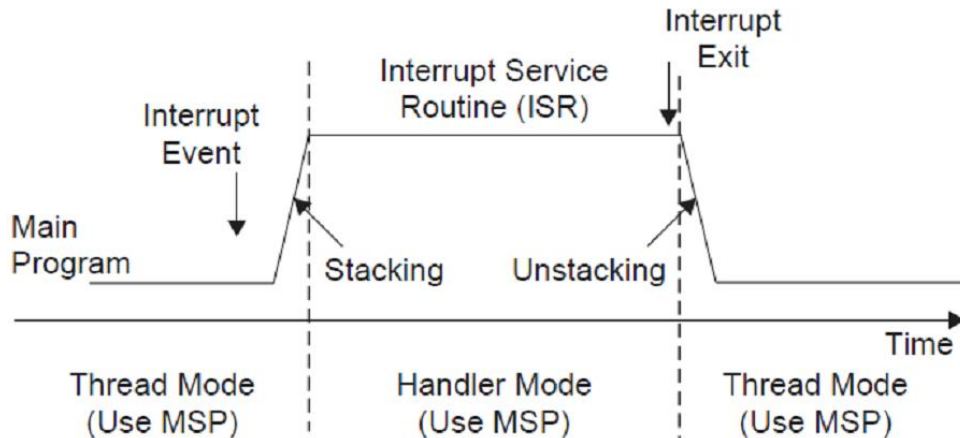
图 2.3.3 CONTROL[1]=0 时的堆栈使用情况
