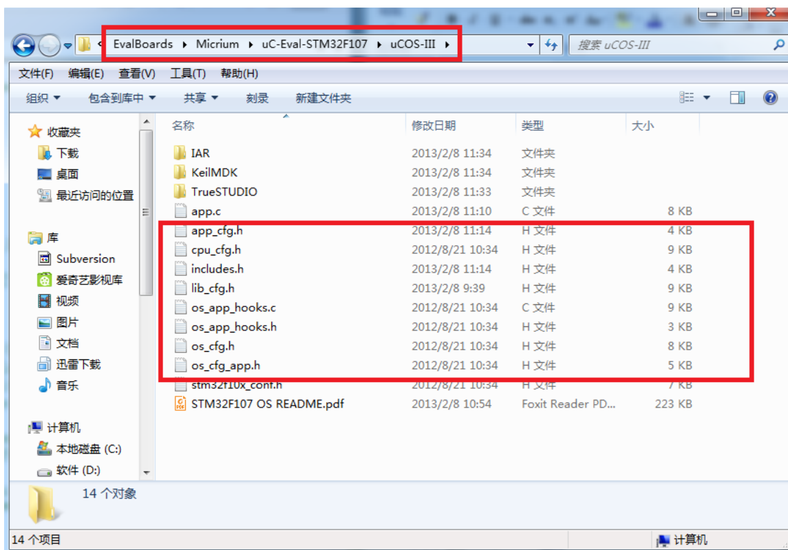
图 4.2.5 EvalBoards 文件
