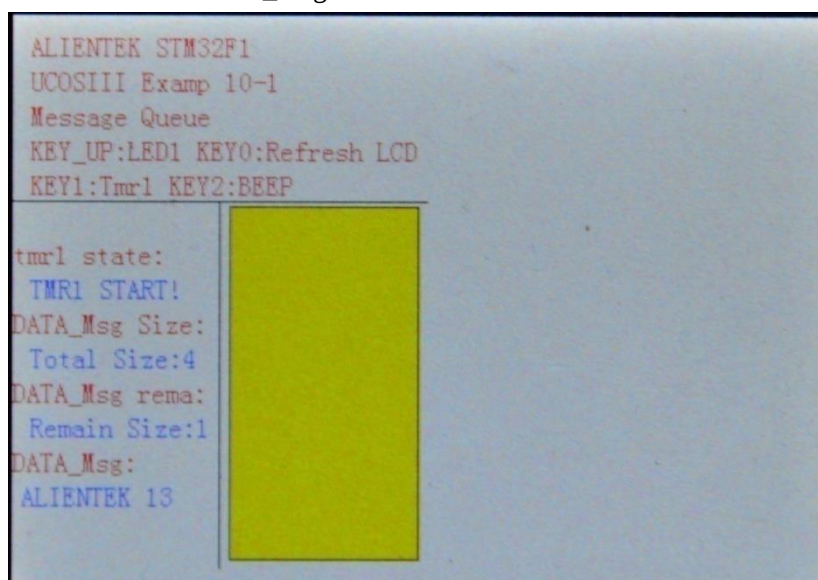
图 10.3.3 开启定时器 1
