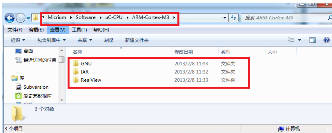
图 4.2.6 ARM-Cortex-M3 文件夹
