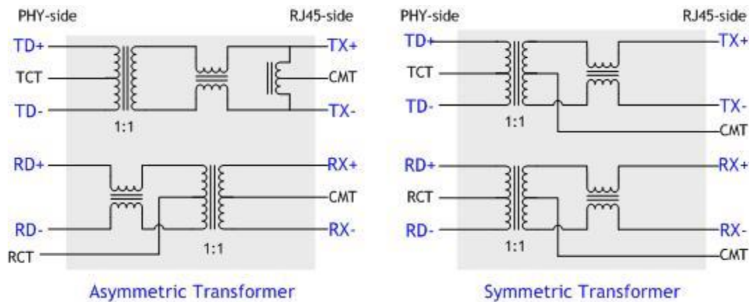
图 24 变压器类型
