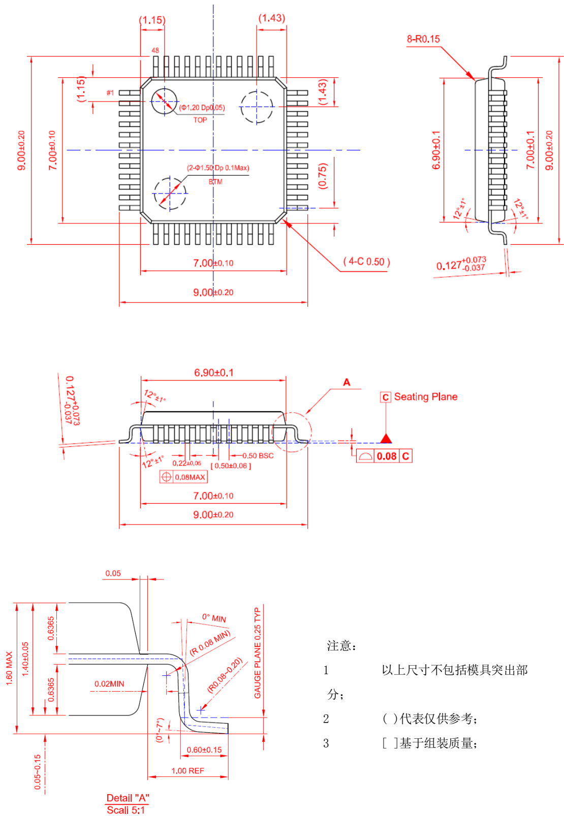
图 25 封装描述
