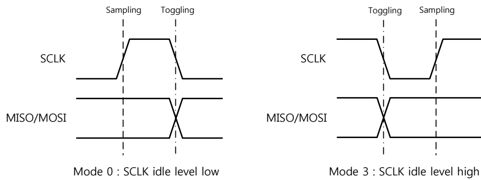
图 6 SPI 模式 0 和 3
