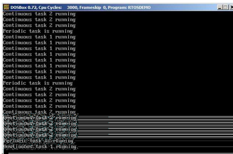
图 11 例 6 的执行输出结果 1
