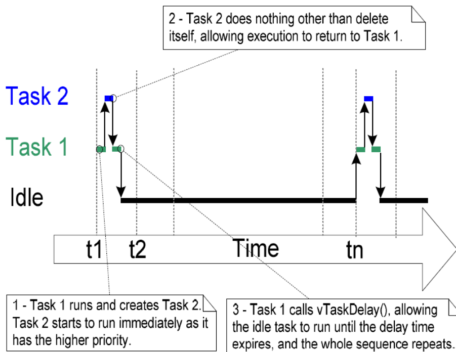
图 17 例 9 执行流程
