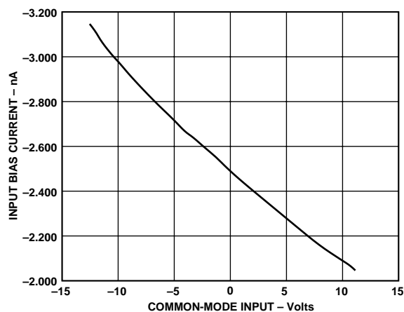
Figure 4. I_{BIAS} vs. CMV, V_S = \pm 15\text{ V} 输入偏置电流与共模输入电压的关系
