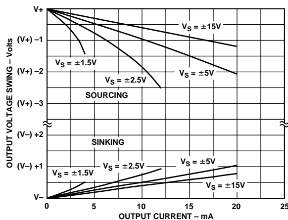
Figure 7. Output Voltage Swing vs. Output Current 输出电压摆幅与输出电流的关系
