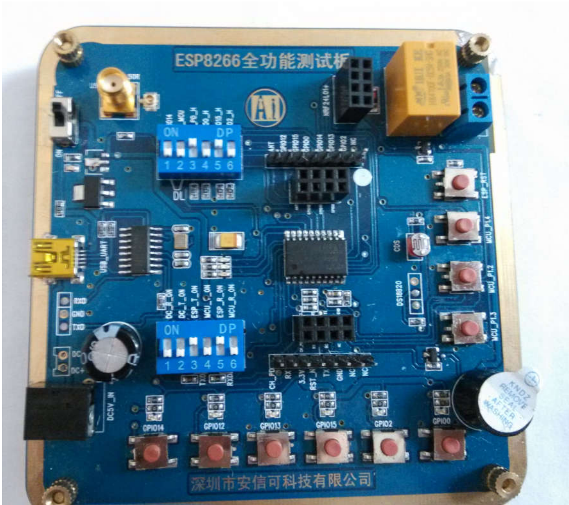
图 6 全功能测试板板正面视图
