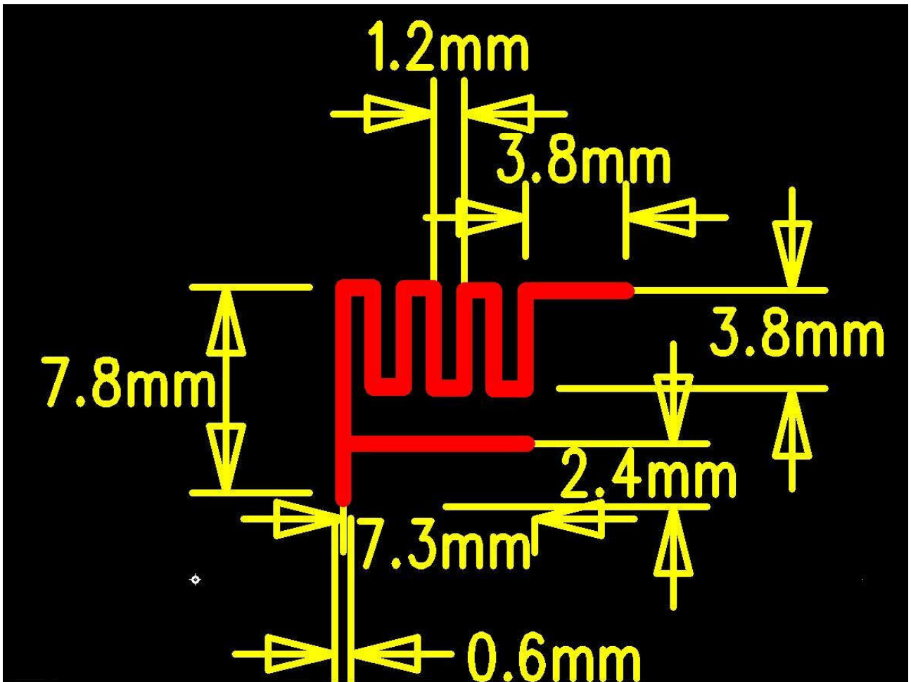
图 3 天线图
