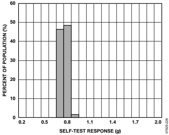
图28 25 °C时的X轴自测响应, V_s = 2.5 V
