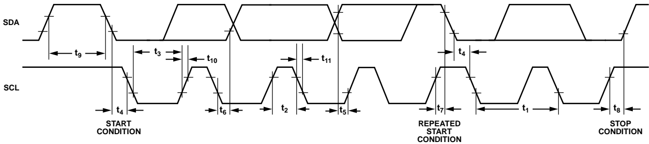
图41. I 2 C时序图
