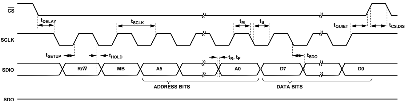
图38. 3线式SPI读取/写入
