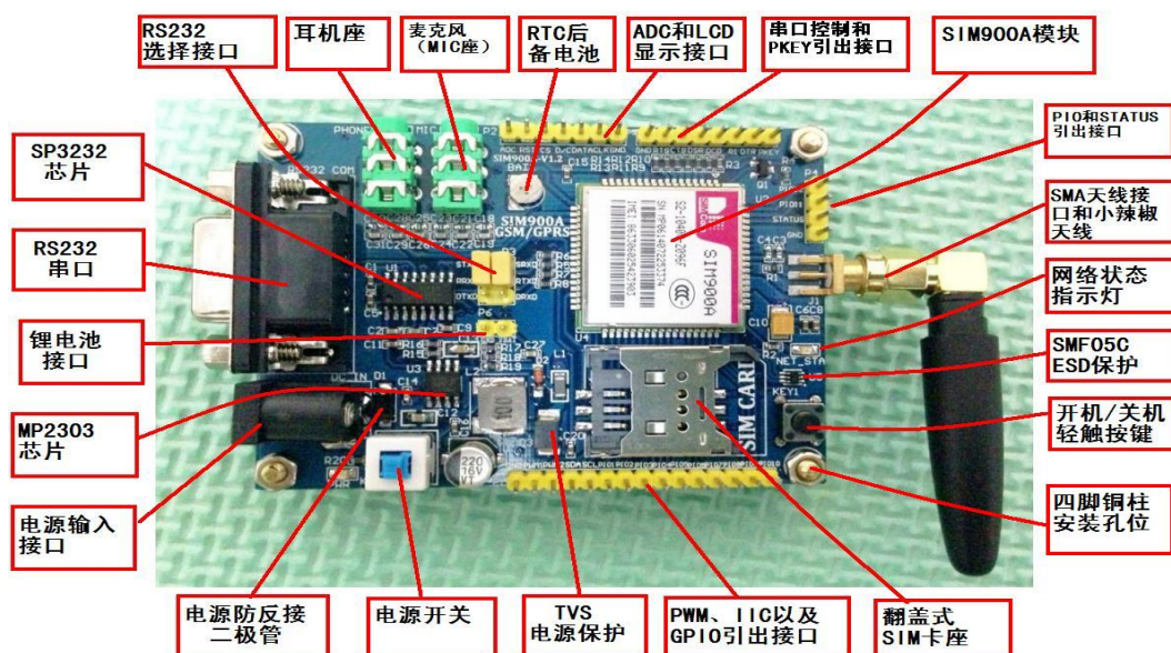
图 1.1.1 ATK-SIM900A 模块资源图
