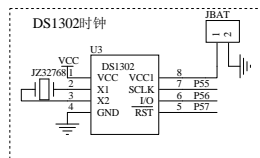
伯乐电子 MSP430F149-V1.2原理图
