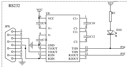
伯乐电子 MSP430F149-V1.2原理图
