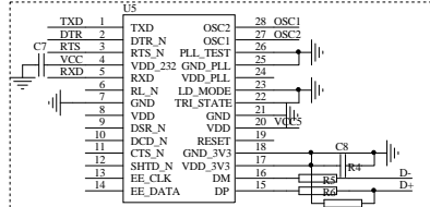
伯乐电子 MSP430F149-V1.2原理图
