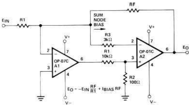
图 8 高速综合放大器
