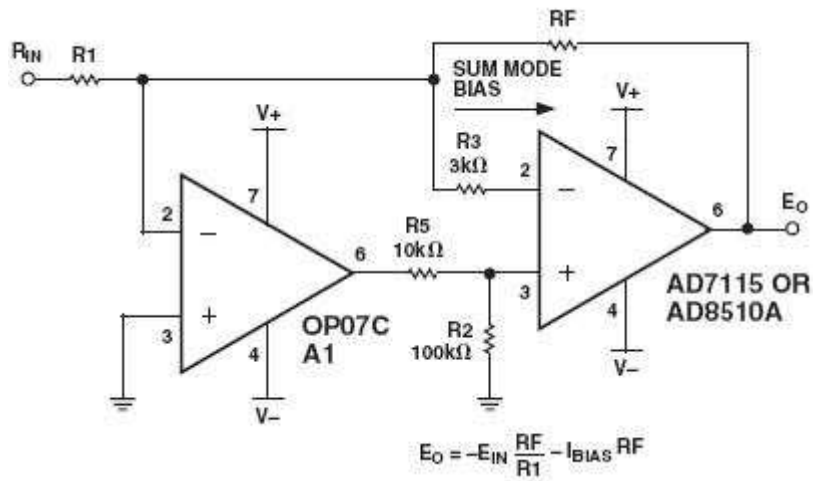
图 5 典型的偏置电压试验电路
