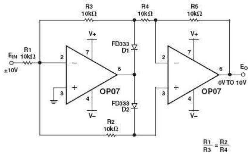
图 6 老化电路
