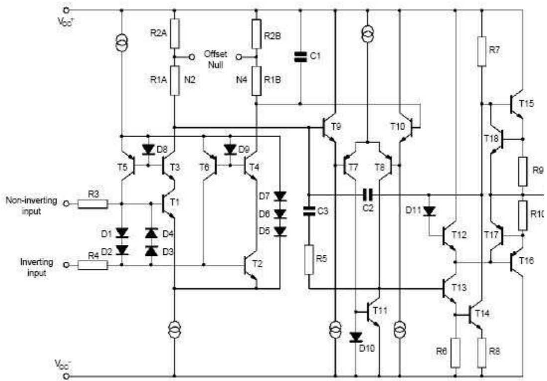
图 3 OP07 内部电路图
