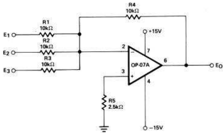
图 10 调整精度放大器
