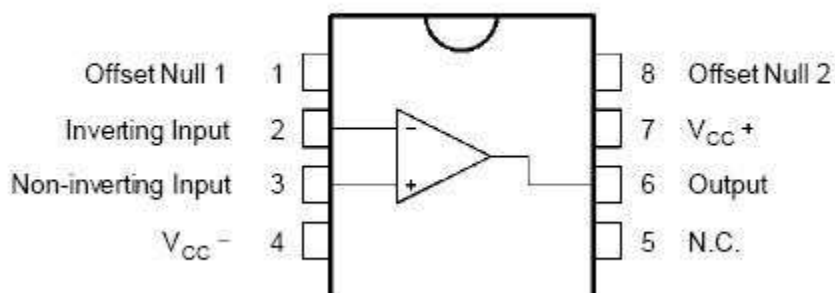
图 2 OP07 管脚图
