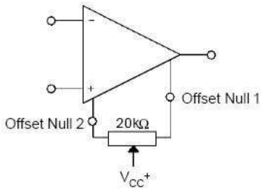
图 4 输入失调电压调零电路
