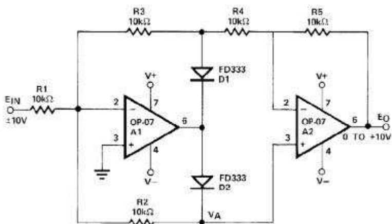
图 12 精密绝对值电路
