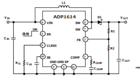
图1. 升压调节器配置
