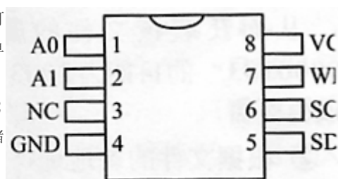
图 1 AT24C512 引脚
