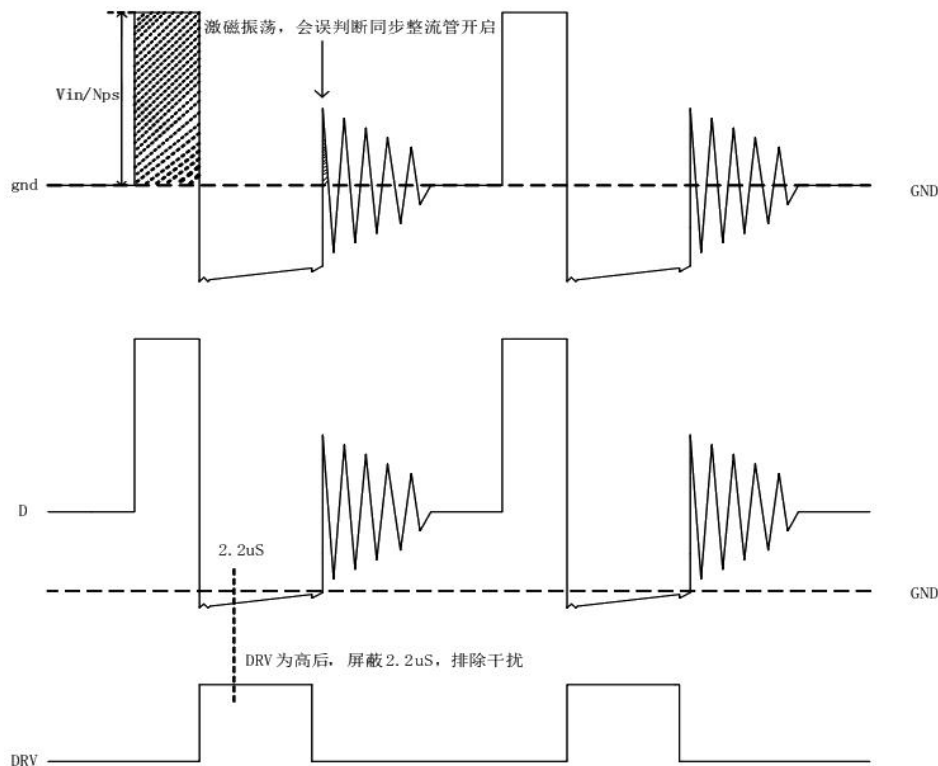
系统关键节点相对于GND波形
