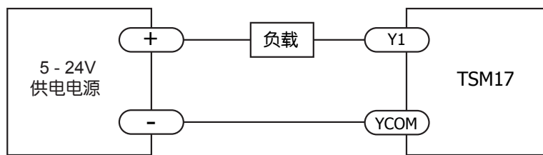
灌电流输出的连接方式
