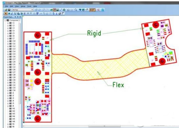
图 4：刚性/柔性电路板允许最大限度地利用可用空间。
