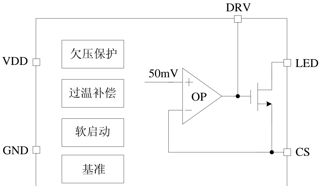
图 2: QX7136 的内部电路方框图
