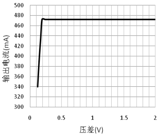
输出电流与压差特性曲线
