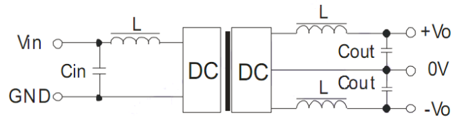
双路输出
