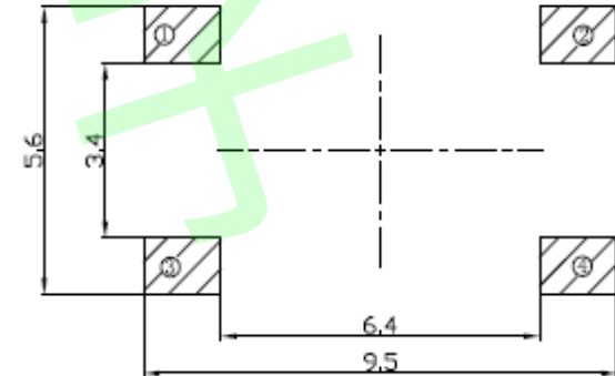
安装参考图
