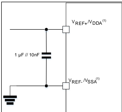
图 52. 供电电源和参考电源去藕线路( V_{REF+} 与 V_{DDA} 相连)
