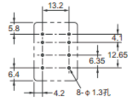
印刷电路板加工尺寸
