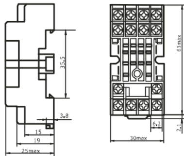
外形图
