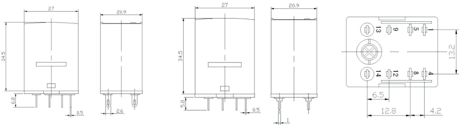
<外形图-插入式>
