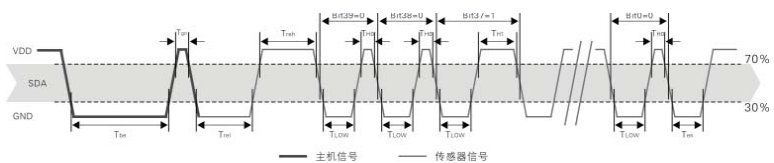
图8: AM2120单总线通信时序
