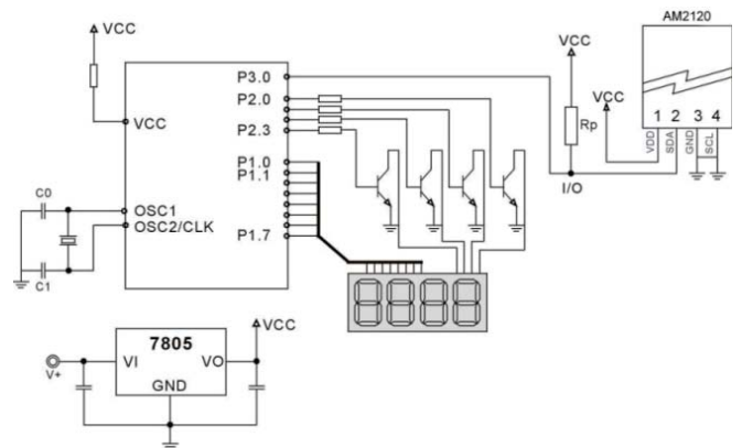
图6: AM2120单总线典型电路
