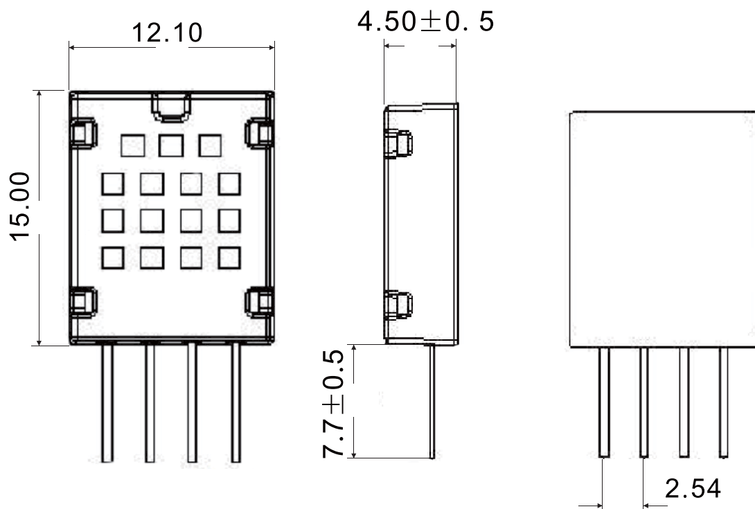
图 1: AM2120 传感器封装图(单位: mm 未注明公差: 0.1mm)
