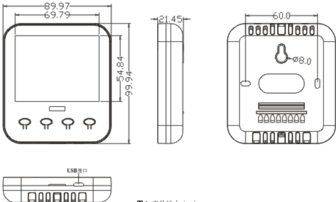
图1 产品尺寸 (mm)
