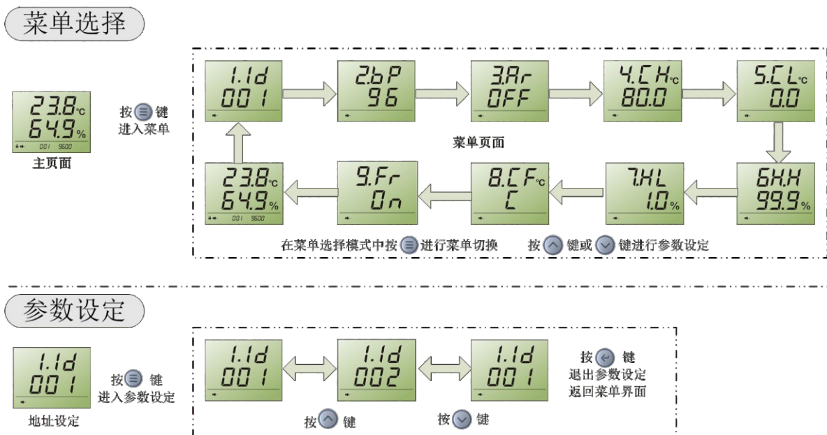
图6 菜单设置演示说明图
