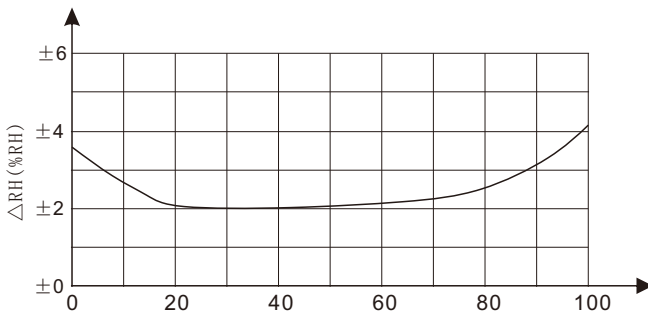
图 8 25°C 不同时间段的湿度误差图
