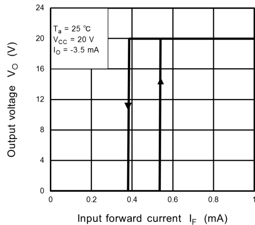
Fig. 12.2.4 V_O - I_F(I_{HYS})
