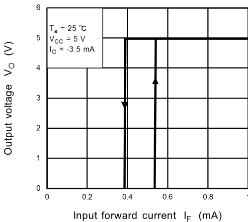
Fig. 12.2.3 V_O - I_F(I_{HYS})
