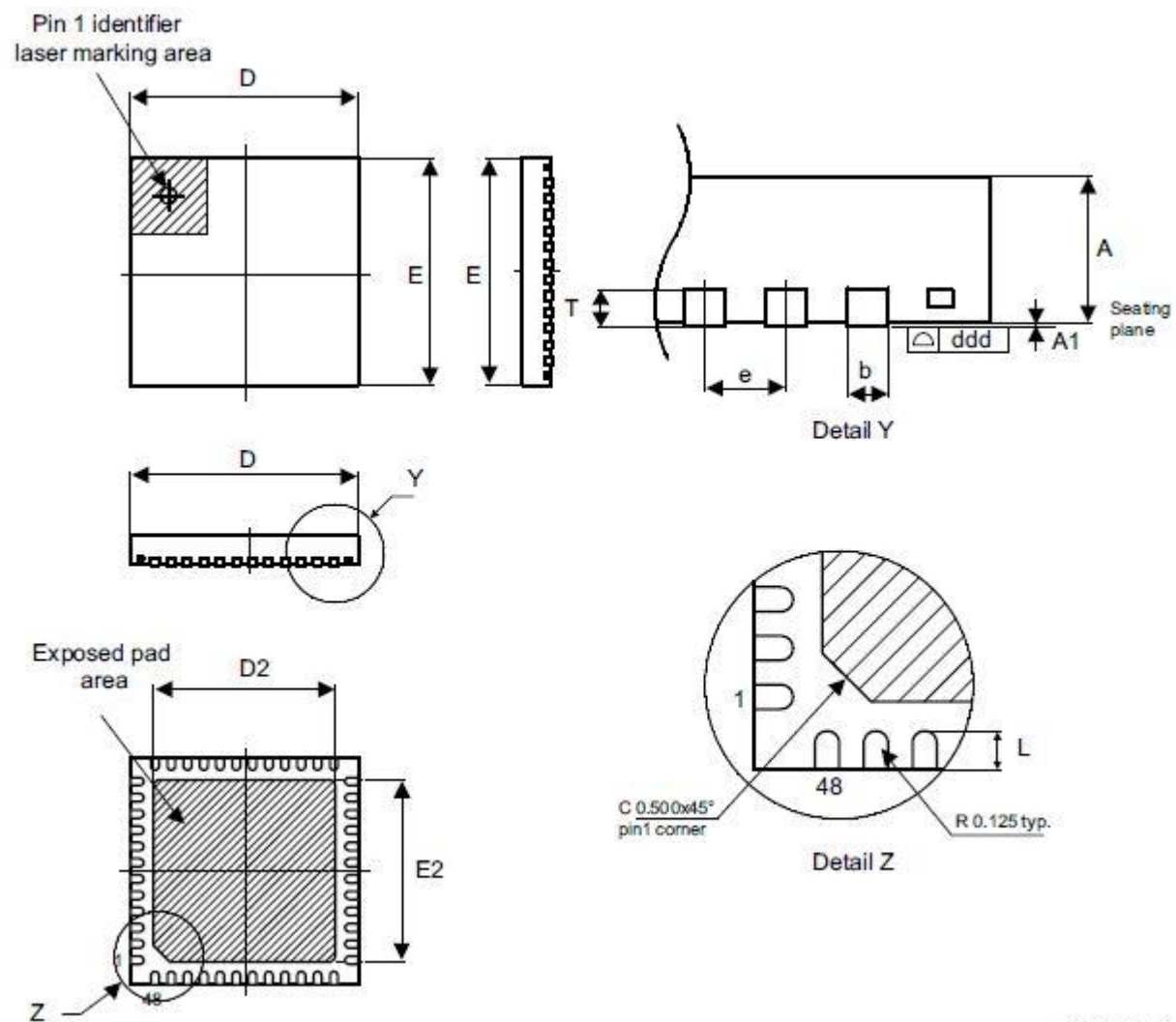
图 35 UFQFPN48 封装外形 (1)
