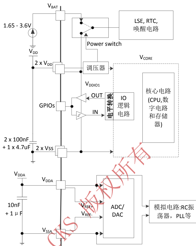
图 11 供电方案
