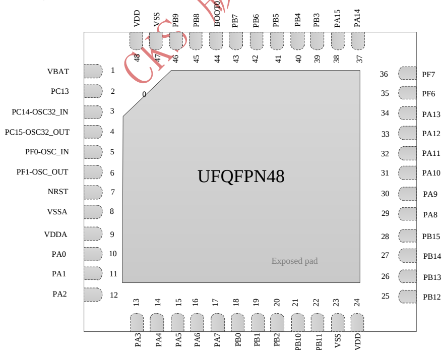
图 5 UFQFPN48 脚封装脚位
