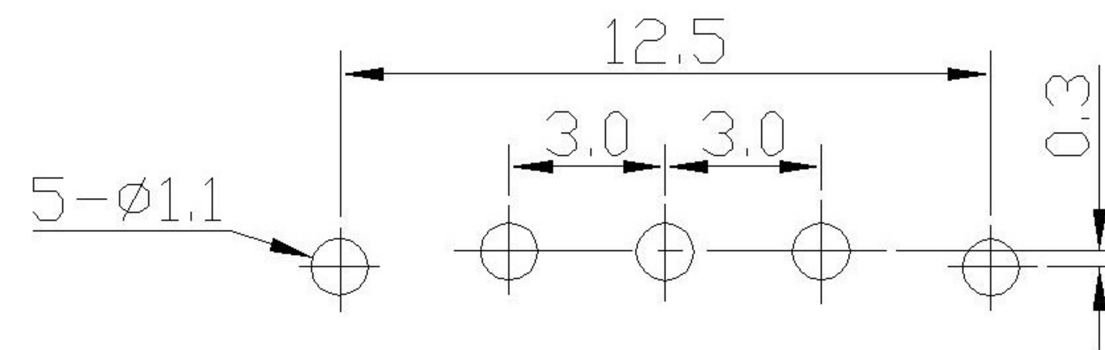
P.C.B LAYOUT
