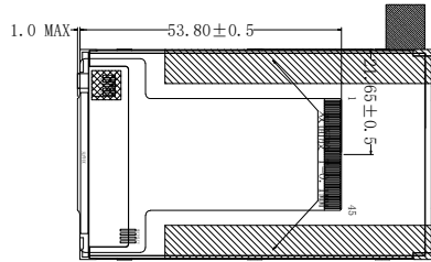
FPC展开示意图
