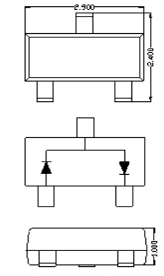
SOT23
