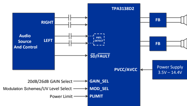
简化原理图
