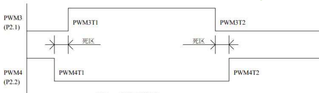
图2: 死区说明
