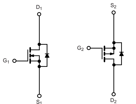
P-Channel MOSFET
