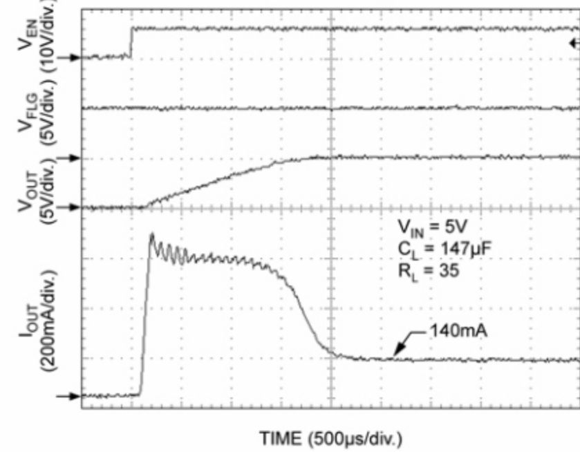
Turn-On ( XL2026-1)
