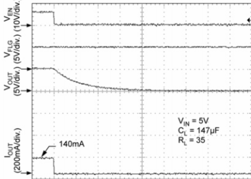
Turn-Off ( XL2026-1)
