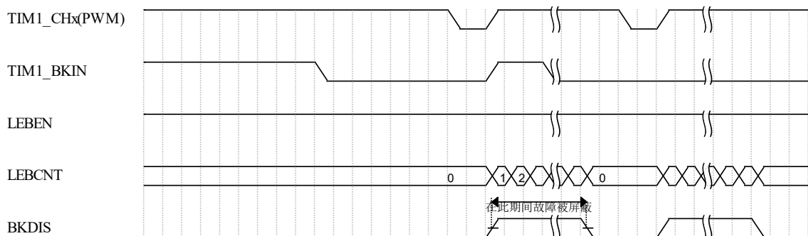
图 10.41 前沿消隐时序示意图
