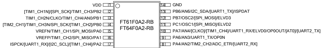
图 1.4 SOP14 脚位
