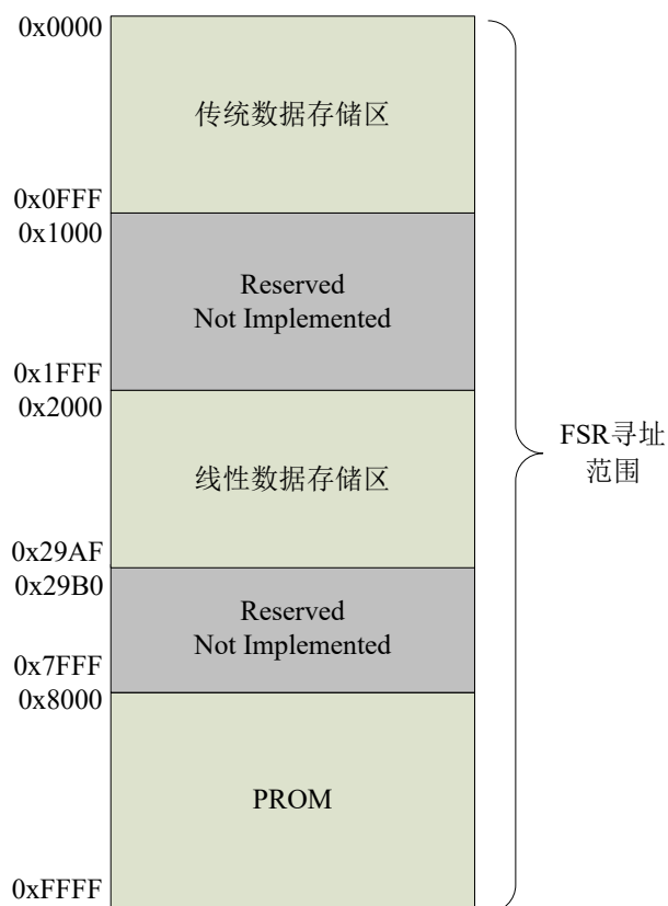
图 3.4 间接寻址
