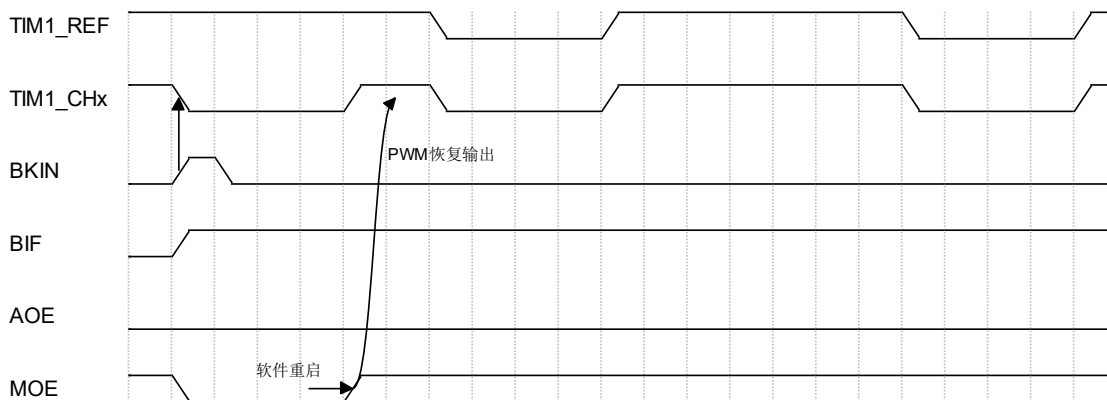
图 10.38 PWM 的自动重启
