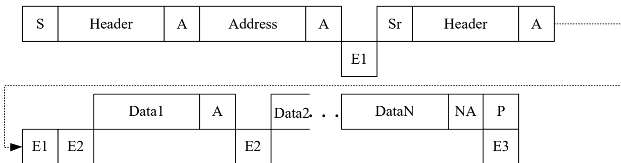
图 14.7 10 比特地址模式从机发送流程图
