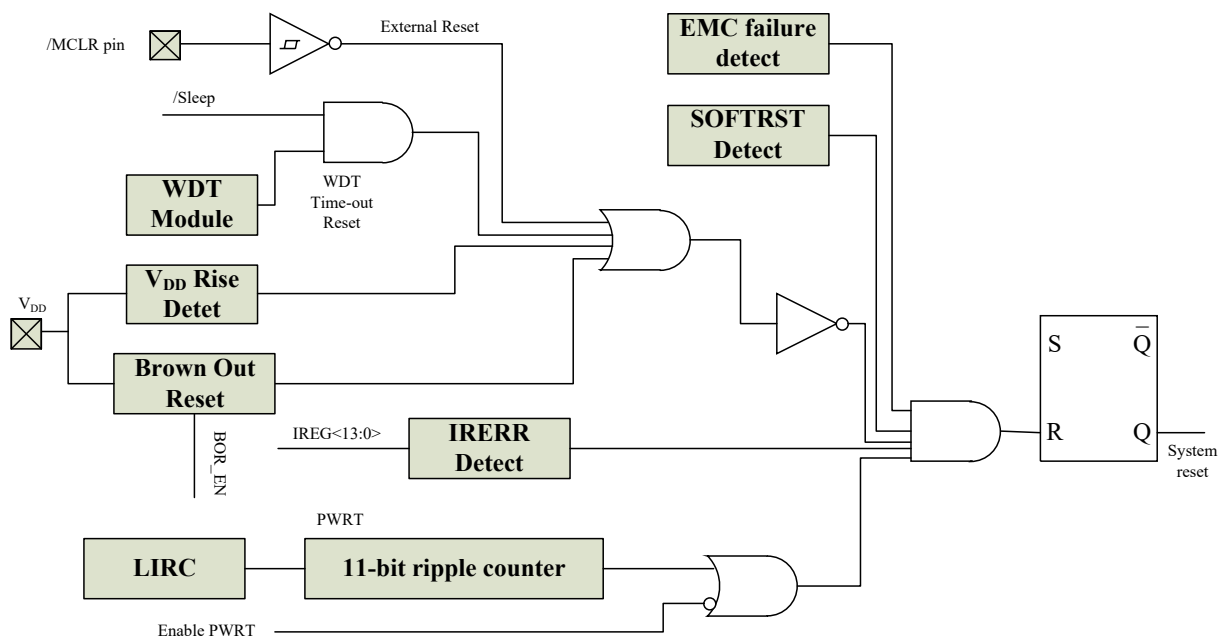
图 4.1 复位框图
