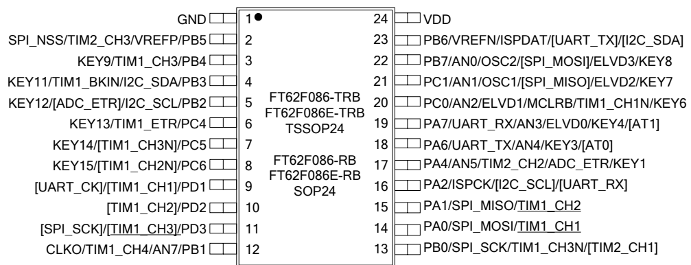
图 1.5 SOP24/TSSOP24 脚位
