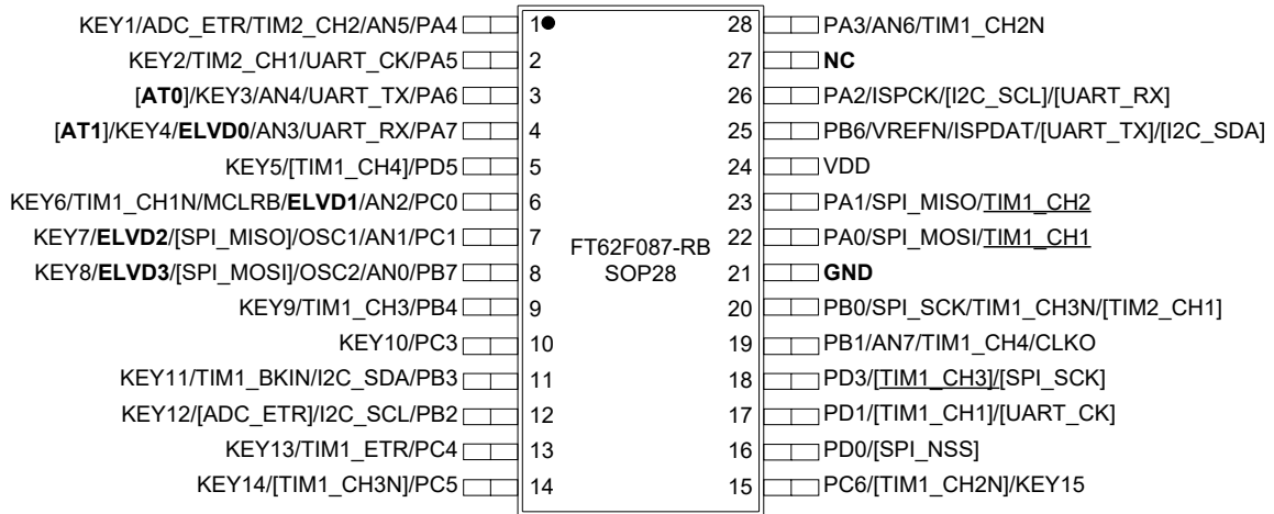
图 1.6 SOP28 脚位
