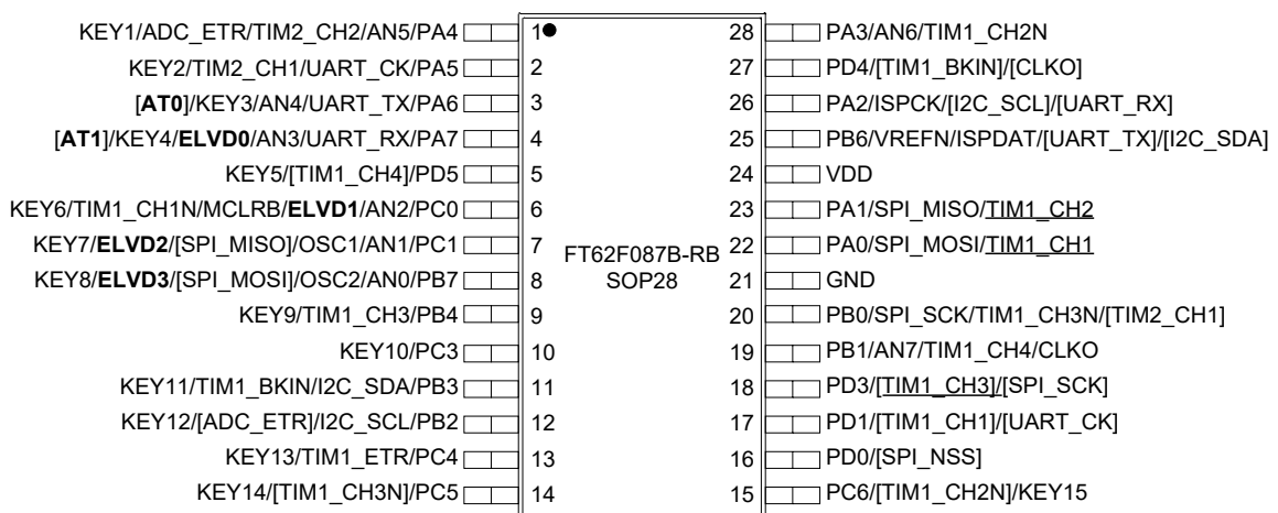
图 1.8 SOP28 脚位 B
