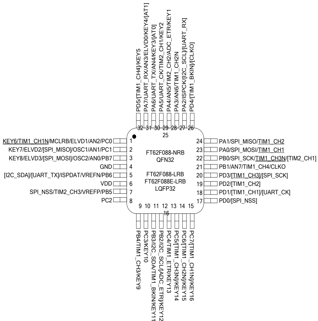
图 1.10 LQFP32/QFN32 脚位
