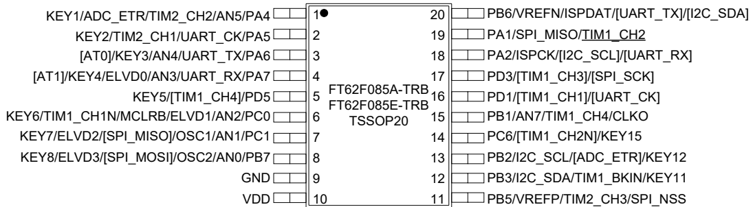
图 1.3 TSSOP20 脚位
