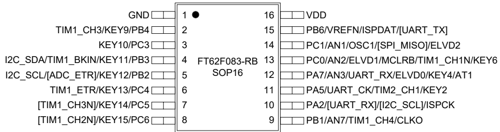
图 1.2 SOP16 脚位
