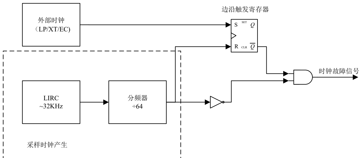
图 5.4 FSCM 原理框图
