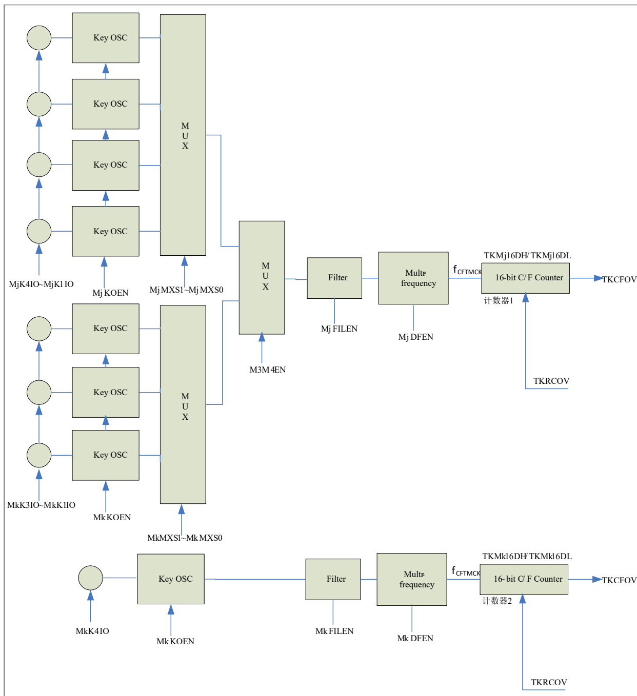
第 2 组触控按键功能方框图 (j=2 k=3)
