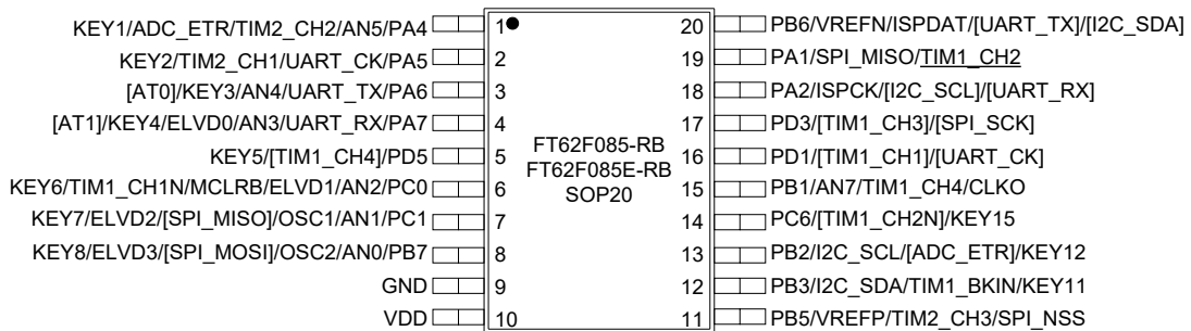
图 1.4 SOP20 脚位
