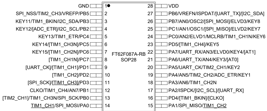
图 1.7 SOP28 脚位 A
