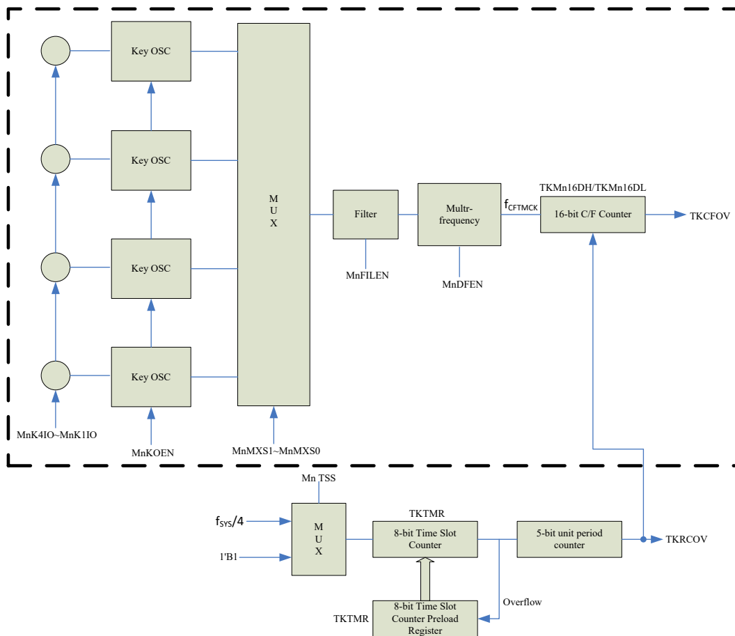
第 1 组触控按键功能方框图 (n=0, 1)
