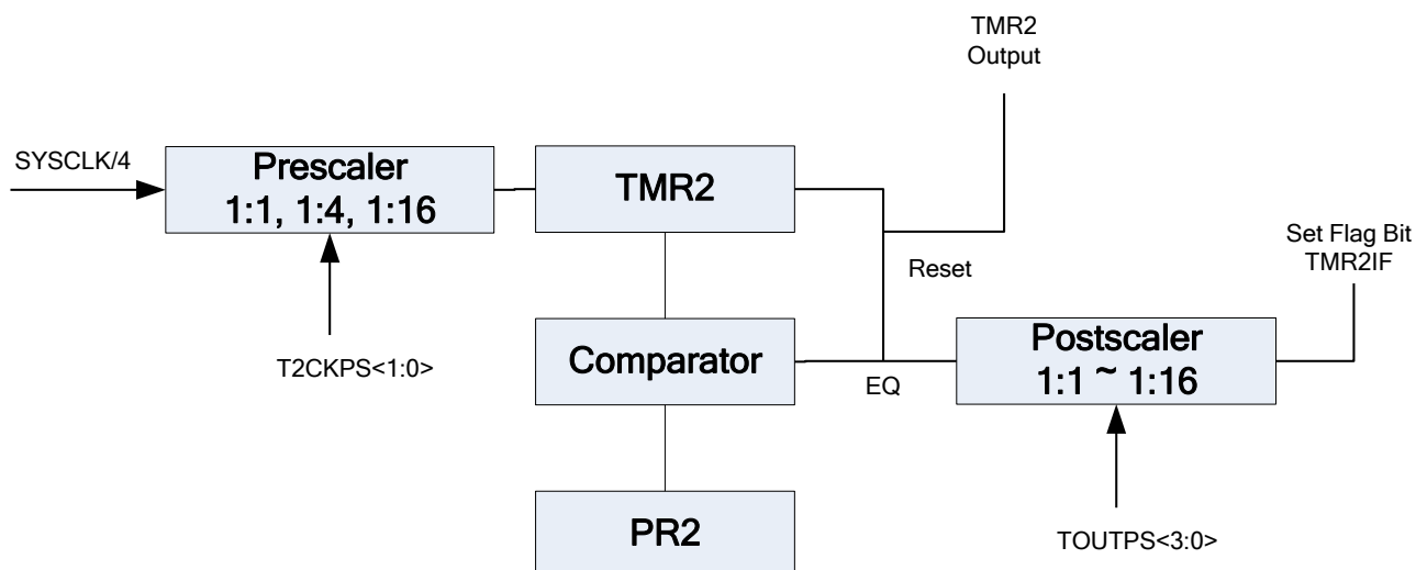
图 9.1 定时器 2 框图
