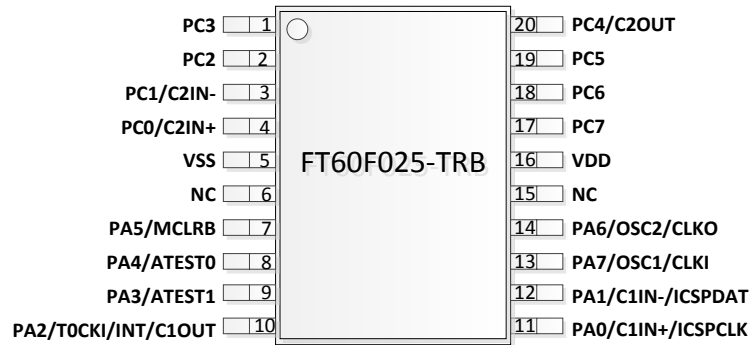
图 1.8 TSSOP-20 脚位图
