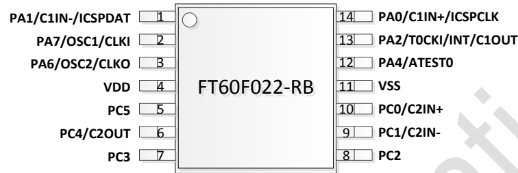
图 1.4 SOP-14 脚位图
