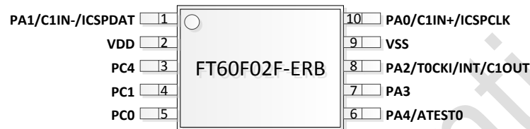
图 1.9 SSOP-10 脚位图
