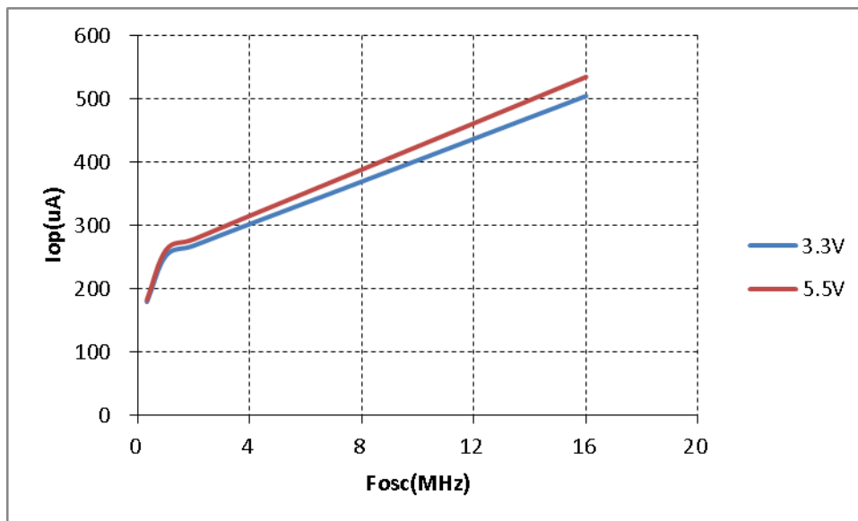
图 16.5 不同 VDD 下芯片工作电流与 Fosc 曲线 ( T=25^{\circ}C )
