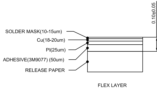
FLEX LAYER
