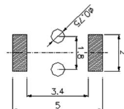
PCB. 焊接图
