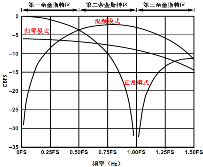
图 38 CBM97D39 在不同模式下 SINC 函数的滚降特性
