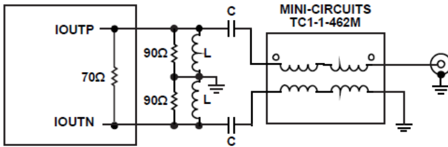
图 46 在混频模式下推荐的接口电路
