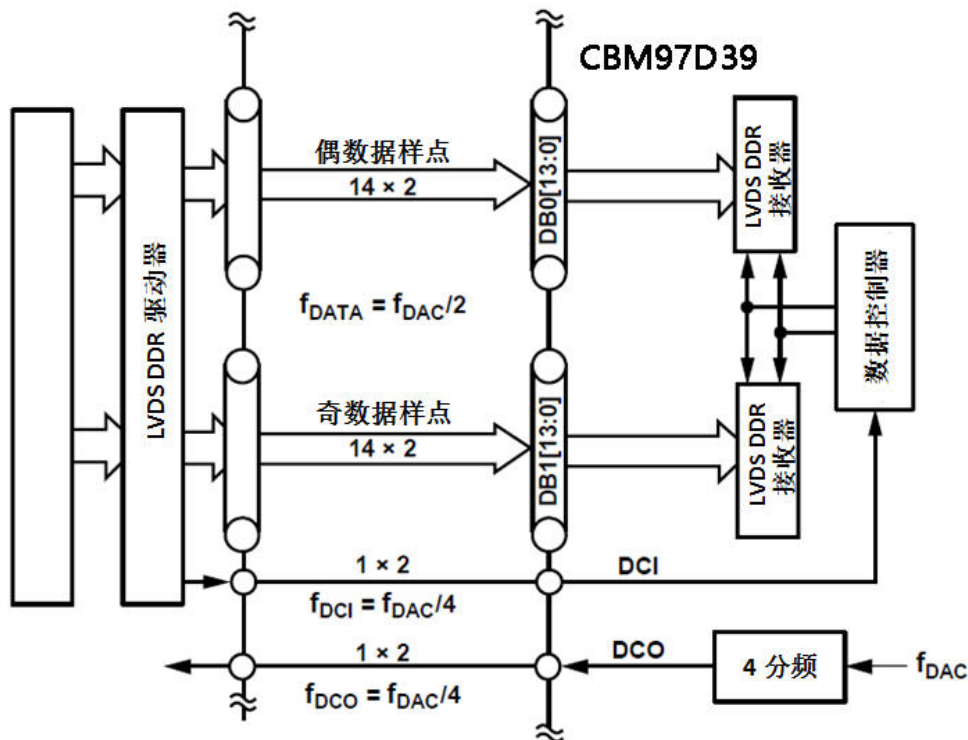
图 23 外部处理器与 CBM97D39 的接口示意图
