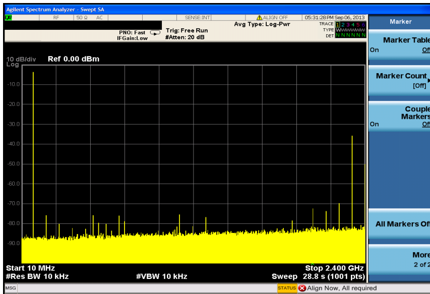
图 3 单音信号频谱, f_{OUT}=91\text{MHz} , f_{DAC}=2.4\text{GSPS}
