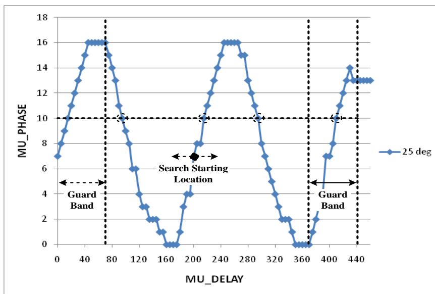
图 30 MU 相位特性与延迟的关系曲线
