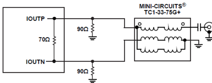
图 44 高达 2.2GHz 输出的推荐电路
