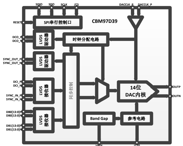
图 1 CBM97D39 功能框图
