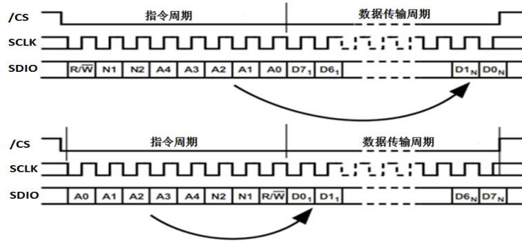
图 19 SPI 串口时序，MSB 优先（上图）和 LSB 优先（下图）
