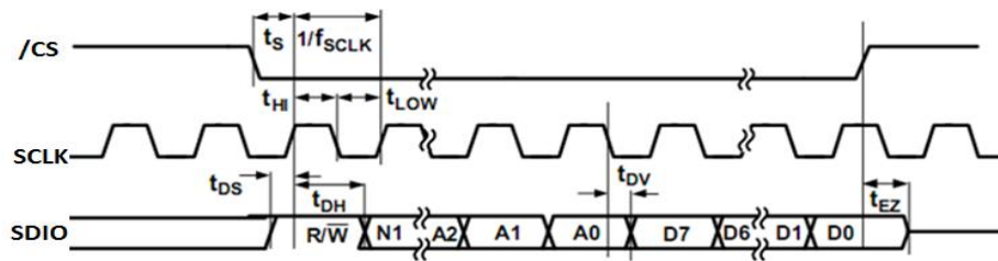
图 21 3 线 SPI 读操作时序
