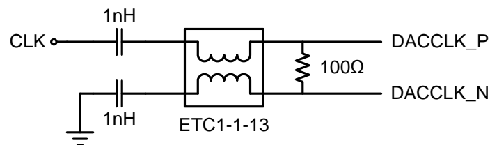
图 39 CBM97D39 的典型时钟输入参考电路
