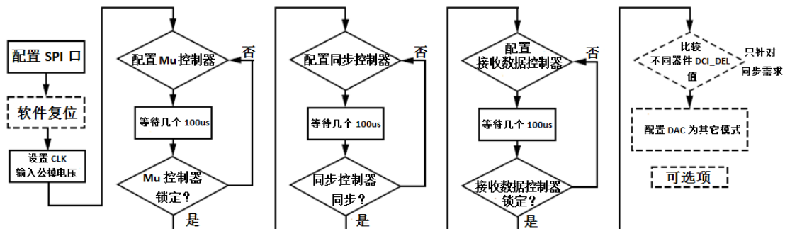
图 47 CBM97D39 的初始化配置流程
