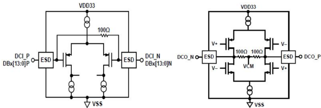
图 27 LVDS 输入和输出等效电路
