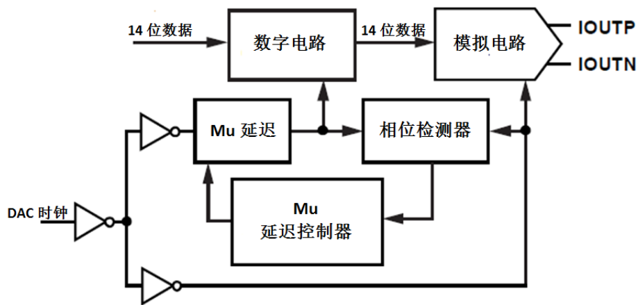
图 29 Mu 延时控制器的框图
