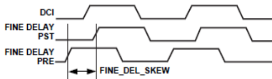
图 26 Pre 延时时钟和 Pst 延时时钟采样图
