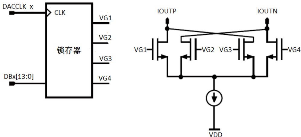
图 35 CBM97D39 的四开关模拟输出架构
