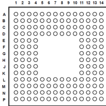
图 2 CBM97D39 管脚图（俯视图，从器件顶部向下看的对应关系）
