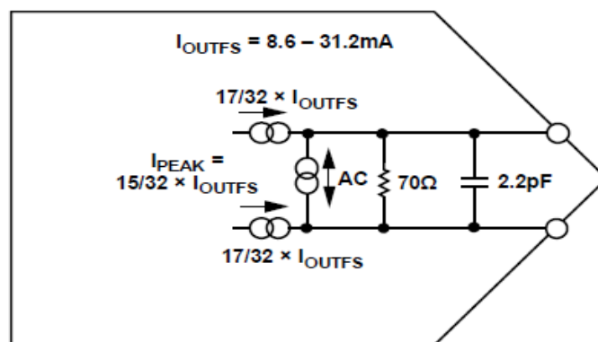
图 41 CBM97D39 的输出等效电路
