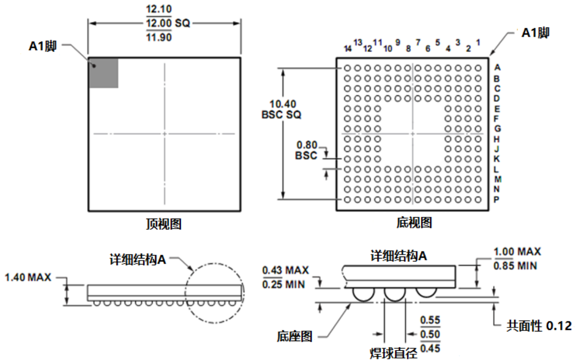
图 48 CBM97D39 外形封装尺寸图
