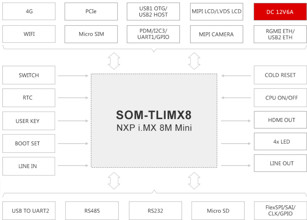
图 5 评估板硬件框图
