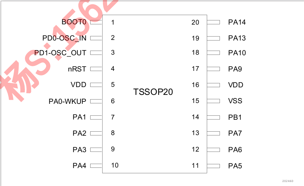
图 8. TSSOP20 引脚分布
