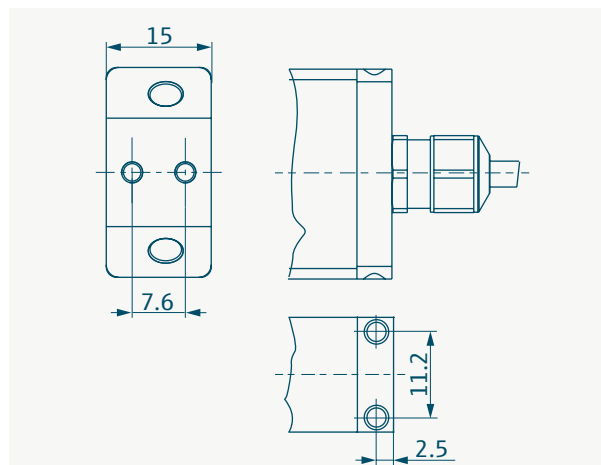
机械固定尺寸，单位为 mm
