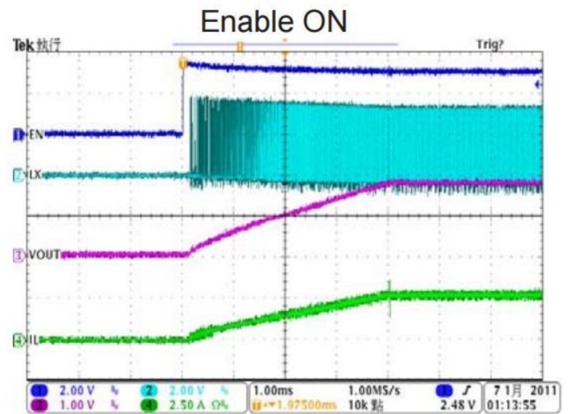
I_{LOAD}: 3A
