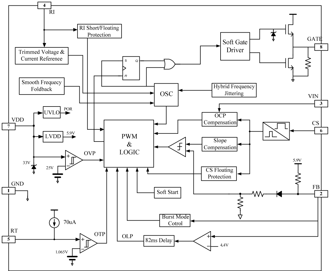
简化内部电路结构图
