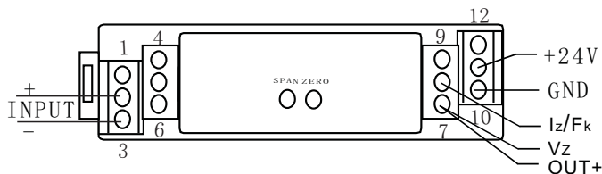
B型变送器接线图(俯视)
