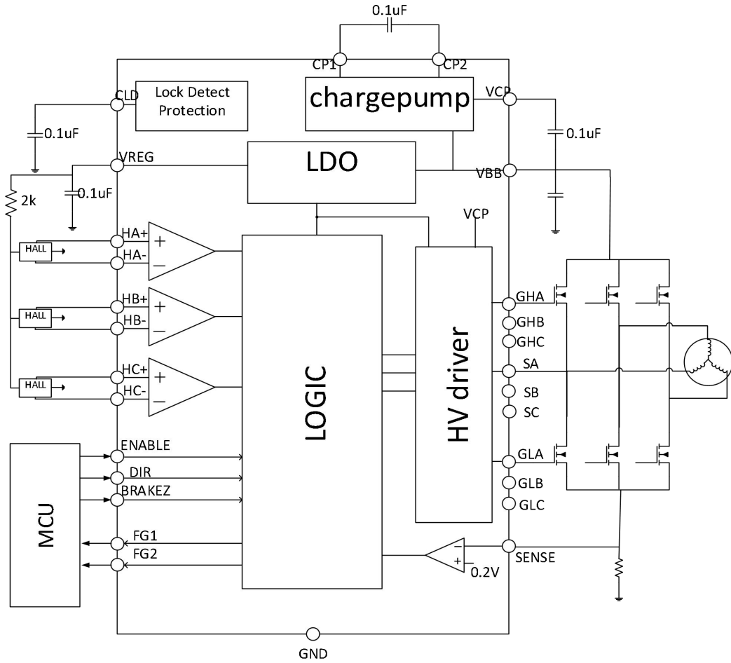
图 4 GC4931 典型应用图
