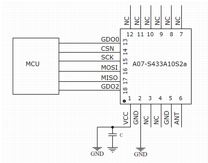
图 5-1 推荐连接图
